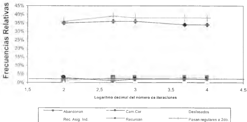
Figura 2. Análisis de Convergencia de las sucesiones generadas por las iteraciones
